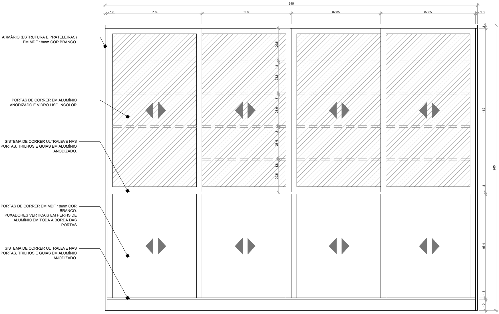
ARMÁRIO GUARDA-VOLUMES - VISTA FRONTAL
